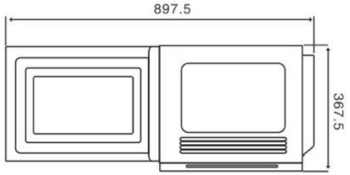
DOOR OPEN
